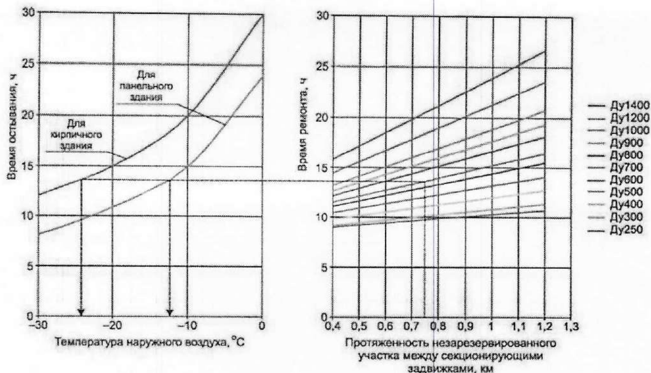
Рис. 7. Номограмма для определения периодов остывания для подъездов и лестничных клеток жилых зданий со снижением температуры с +15 °С до +3°С.
