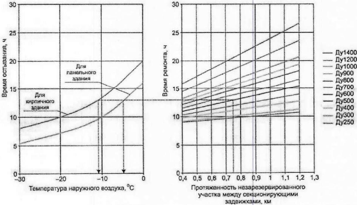
Рис. 6. Номограмма для определения периодов остывания угловых жилых помещений кирпичных и панельных зданий со снижением температуры внутреннего воздуха помещений с +20 °C до +12°C.
